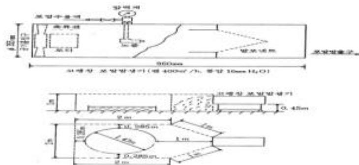
그림 시험장치
